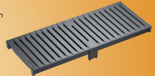
Längsstabrost, Gusseisen D400 & E600 L: 50cm
